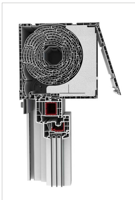
Rewizja tylna RI
