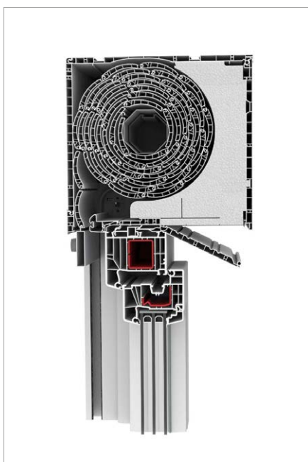
Rewizja dolna RU umożliwia tynkowanie od zewnątrz i od wewnątrz
