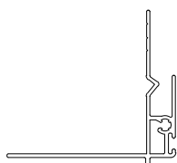
Alu 50 mm | 5451 listwa tynkowa zewn.
